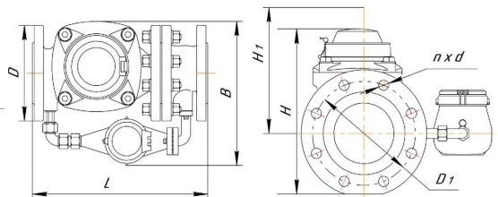
Рис. 2 Размеры счетчика СТБК 2
